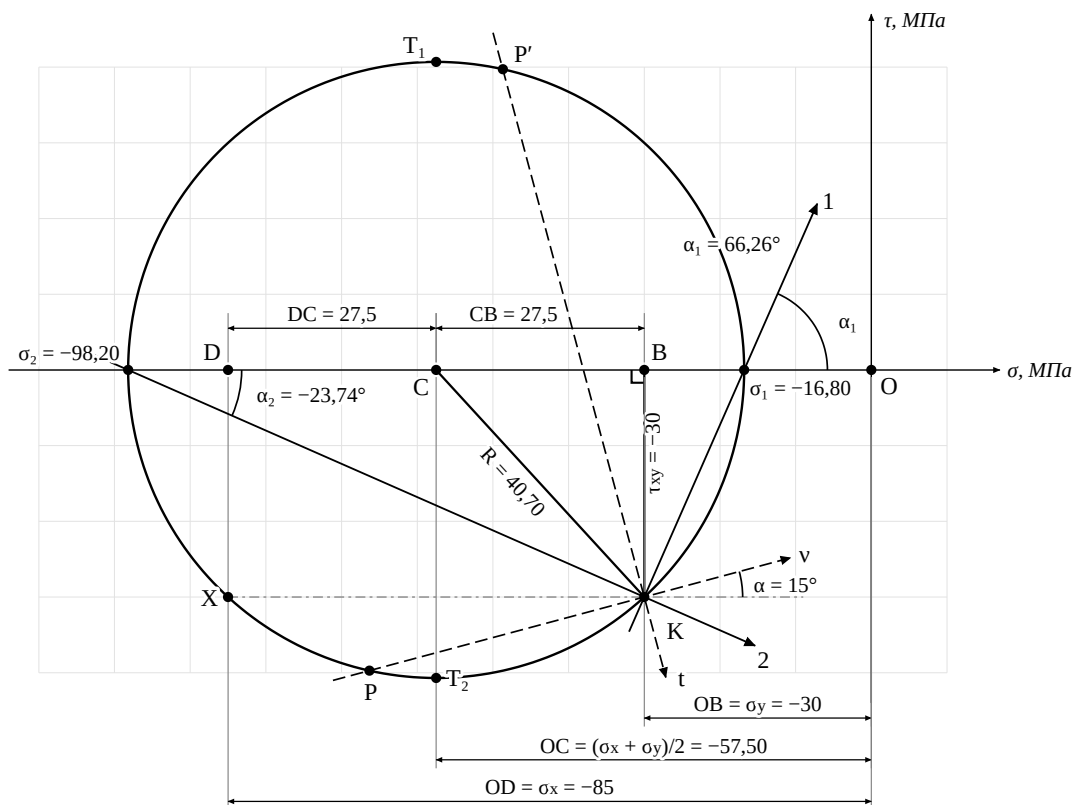
Рис. 7 — круг Мора, 1 см = 10 МПа (сетка — 10 МПа). Лучи 1 и 2 из полюса K — главные направления; T_1, T_2 — \tau_{12} = \pm 40,70 МПа при \sigma' = -57,50 МПа; P и P' — площадки под 15^\circ и 105^\circ : \sigma_v = -66,32 , \tau_{tv} = -39,73 ; \sigma_t = -48,68 МПа.
